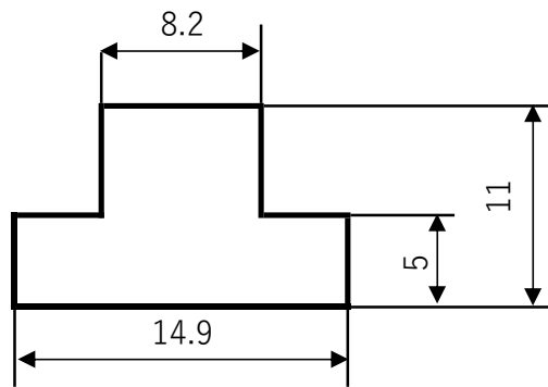
テーブルT溝寸法
