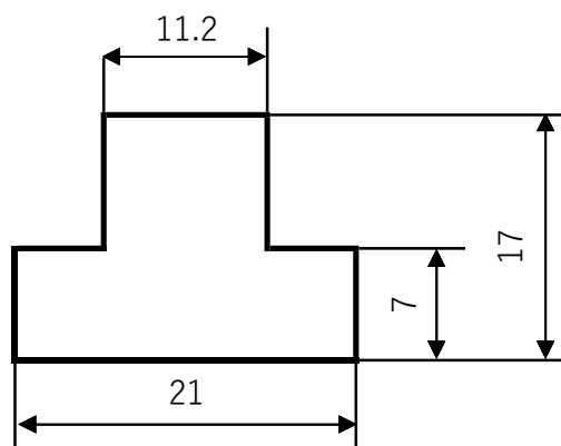
取付Tナット寸法
