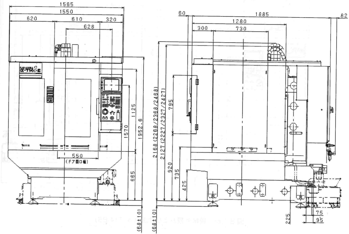
図 B.1(a) 機械外観および寸法 (α-T14iB)
