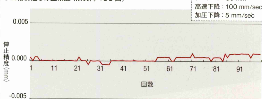
ラム軸繰り返し停止精度 (無負荷 100 回)
