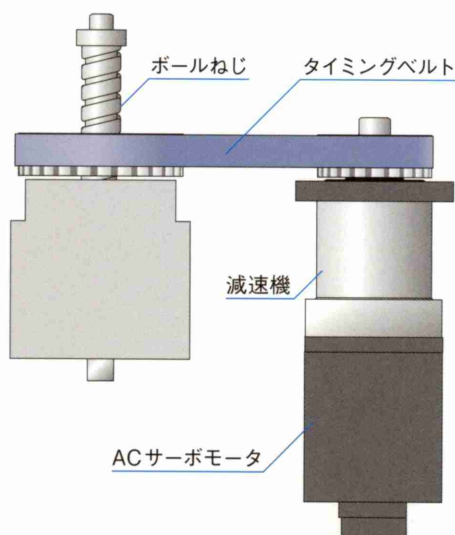
ボールネジ駆動機構
