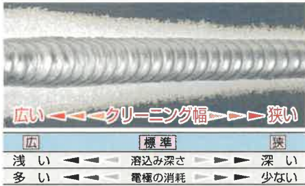
交流TIG溶接(アルミニウム)のクリーニング幅調整機能
