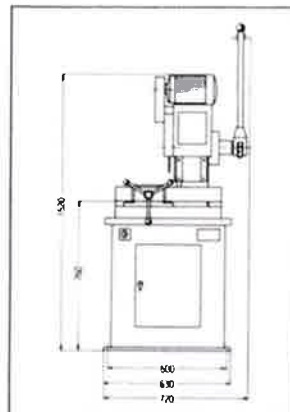
正面図
