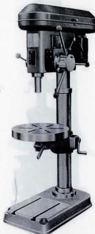
ESD-460 AF 形 自動送り付中型卓上ボール盤
