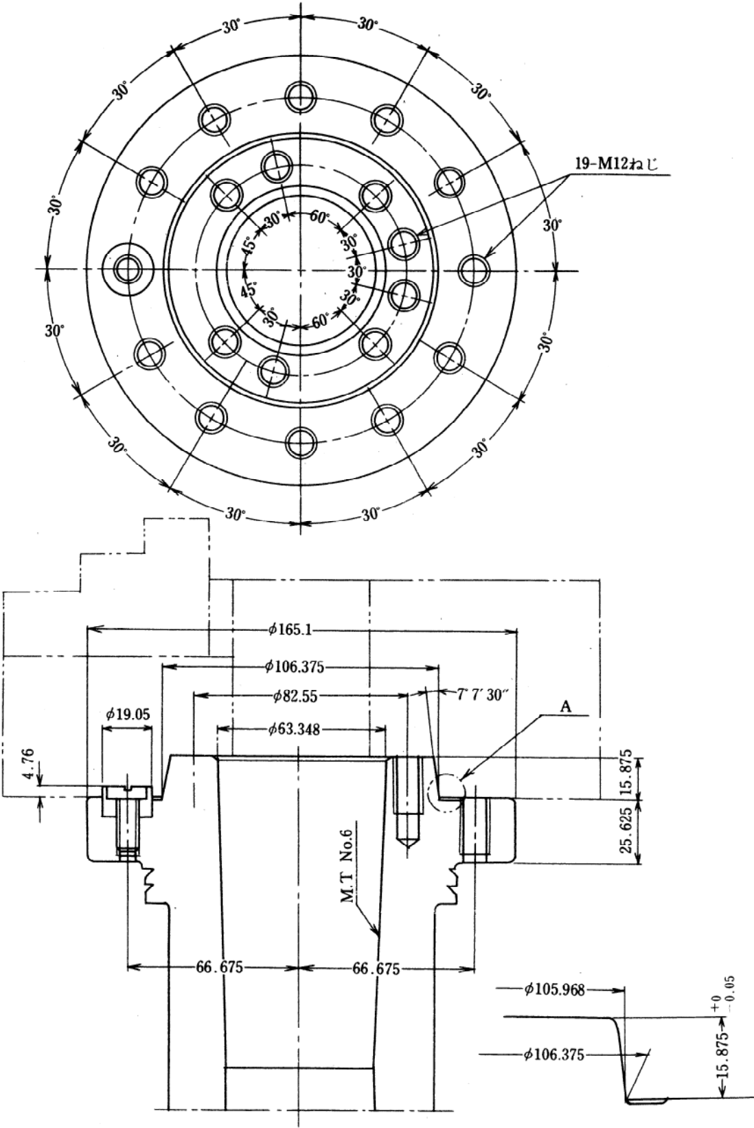
主 軸 端 詳 細 図
