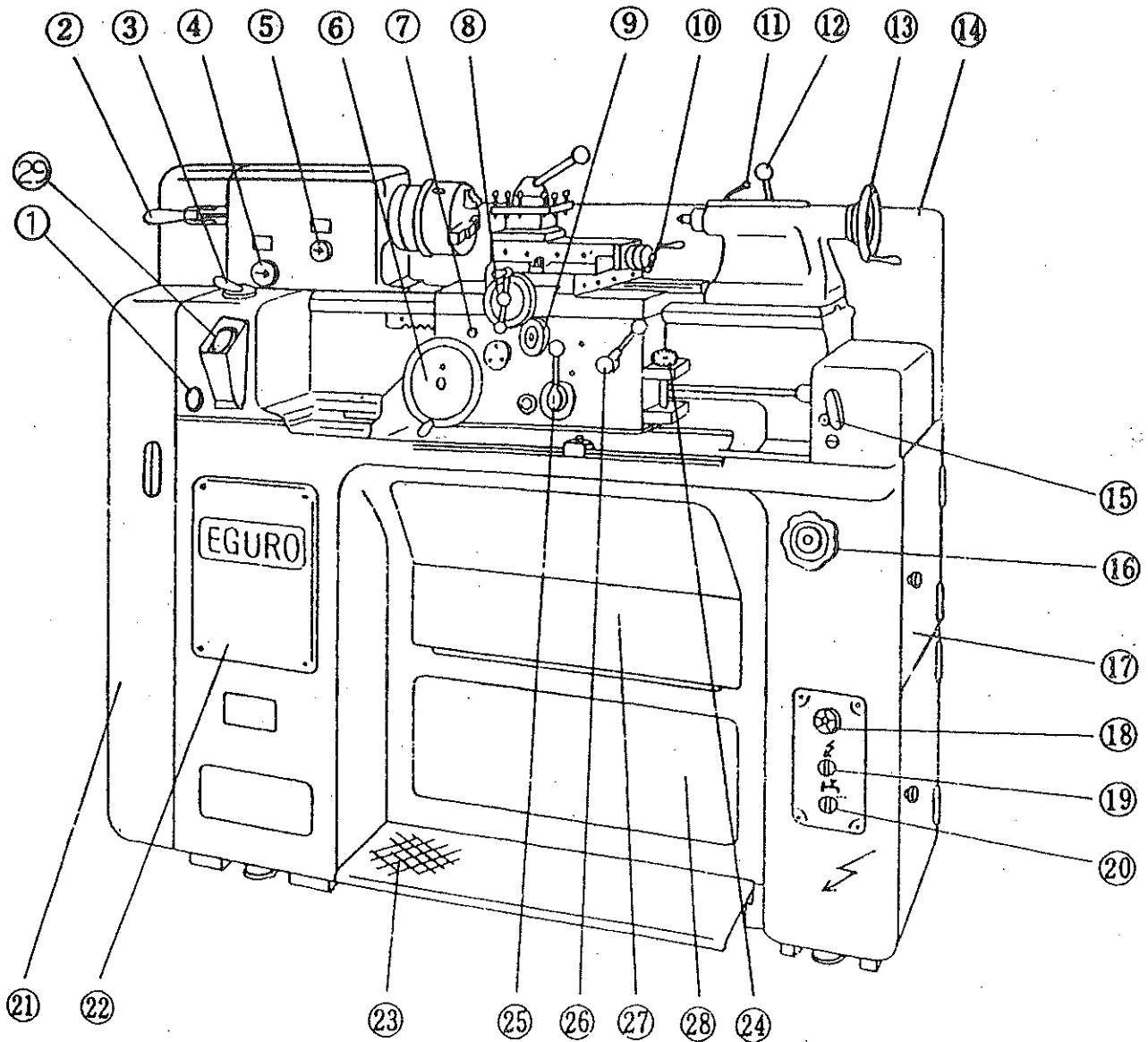
第1図 操作機構図
