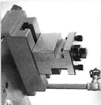
逆バイト台 横送り台面筋の溝により、取付け、取 外しが容易、19mm角または、21mm角の バイトを取付けられます
