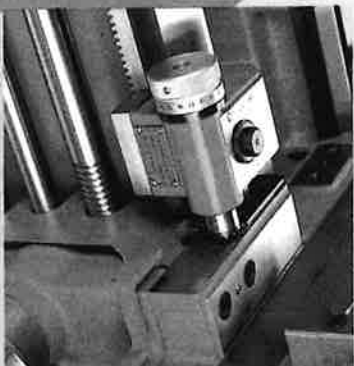
ヘッドストップ ヘッドに取付け、往復台を当てること により長手方向の位置決めをします (ただし、自動送りを停止させることはできません)
