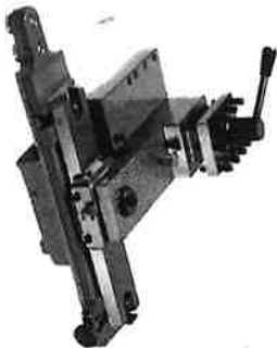
テーパー削り装置 ガイドプレートを用いて容易に テーパー加工ができます。
