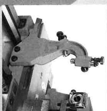
6段ストップバ(MSタイプ) 6本の異なった位置決め棒により、そ れぞれ異なった長手方向の位置決めが 可能です (ただし、自動送りを停止させることはできません)
