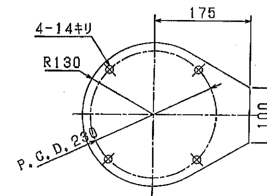
A矢視図 S:1/5
